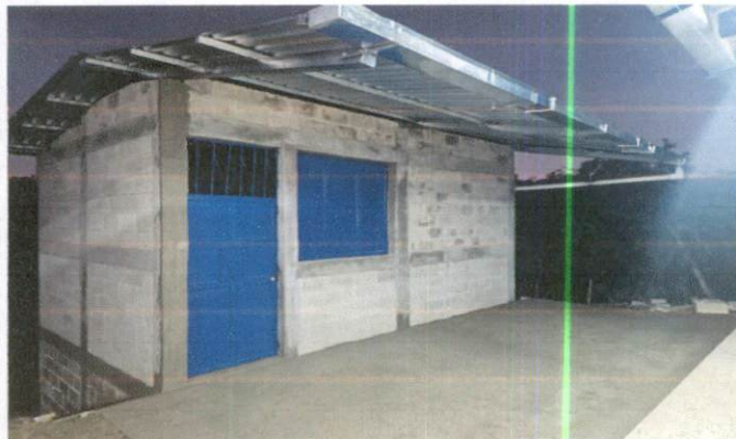
Foto 1: Mejoramiento de techo estructura metálica, láminas troqueladas calibre 26 y tubos cuadrados de 4x4 y 2x2 galvanizado calibre 16, finalizado.
